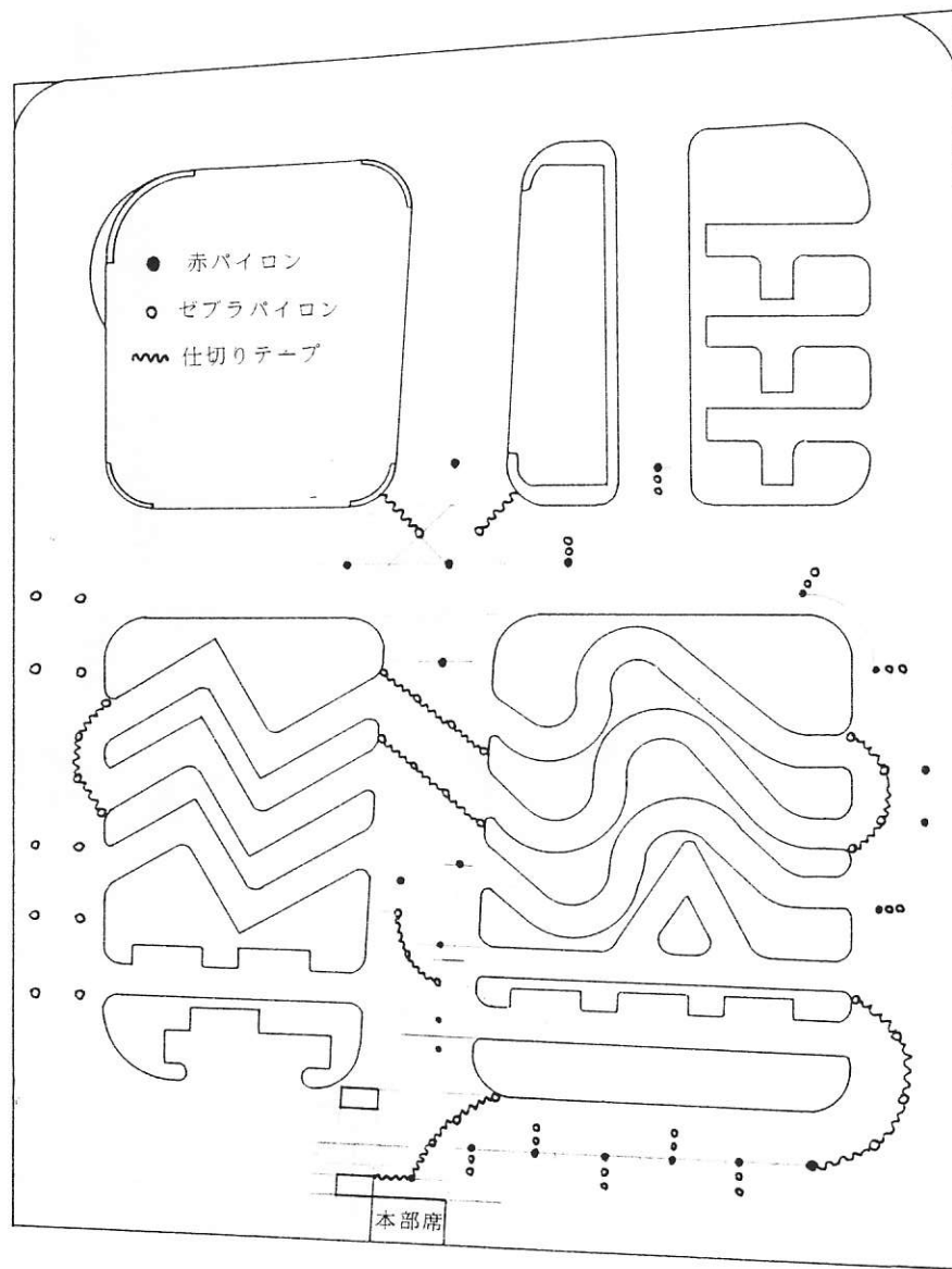
コース作成パイロン、仕切りテープ配置図
